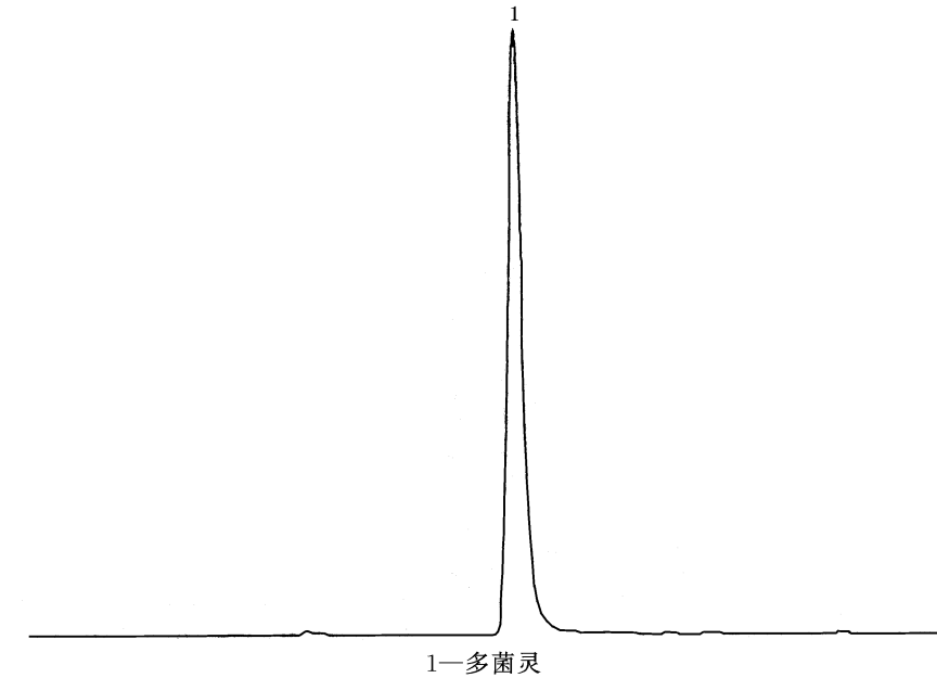
图1 多菌灵原药的高效液相色谱图
